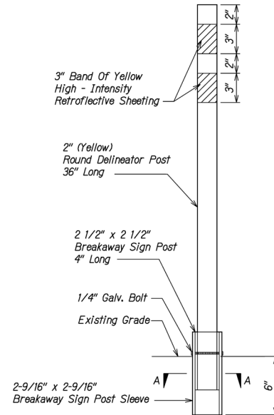
ELEVATION
